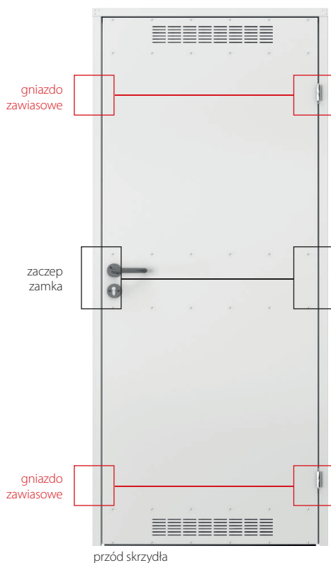
przód skrzydła
